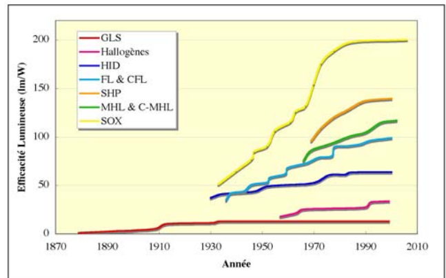
Fig. 4 : Evolution de l'efficacité lumineuse des différentes sources de lumière
