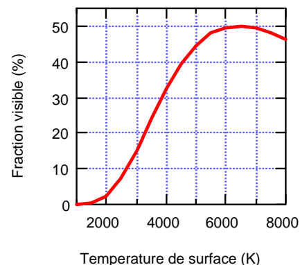
Fig. 5 : Le "poids" du spectre visible dans l'émission totale du corps noir en fonction de la température de sa surface
